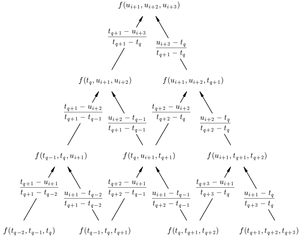
Slika 1.5: Ubacivanje čvorova pomoću Oslo algoritma na primjeru kubičnog splajna
