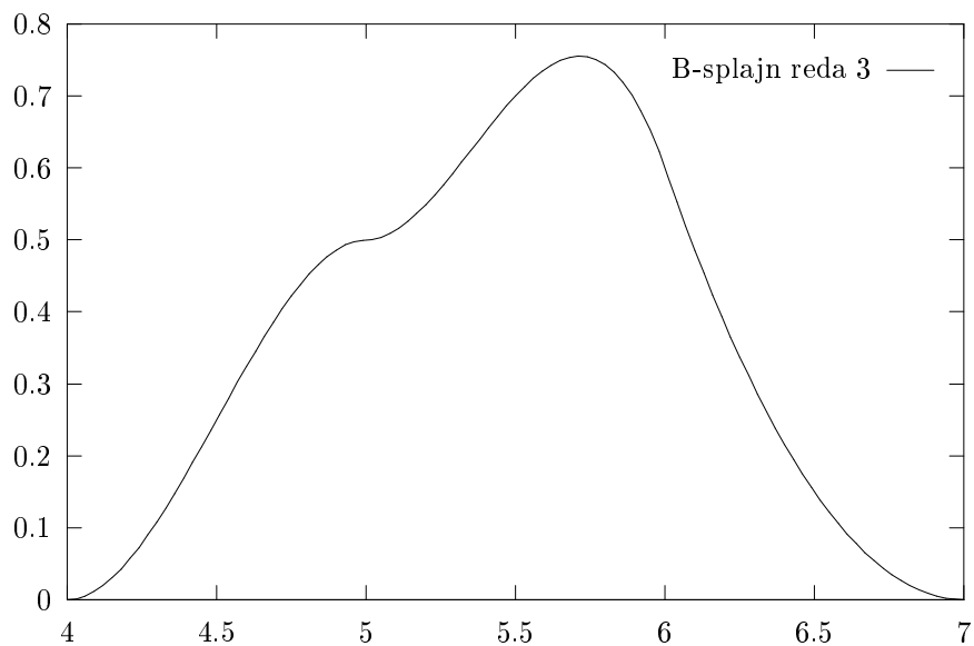
Slika 4.6: B-splajn T_4^3 za q_i = 1, i \neq 5 i q_5 = 0.0001
