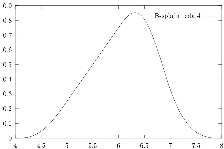
Slika 4.3: B-splajn T_4^4 za q_i = 1, i \neq 5, 6 i q_5 = q_6 = 0.0001
