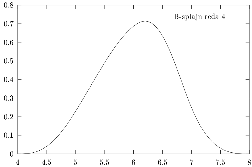
Slika 4.2: B-splajn T_4^4 za q_i = 1, i \neq 5, 6 i q_5 = q_6 = 0.1
