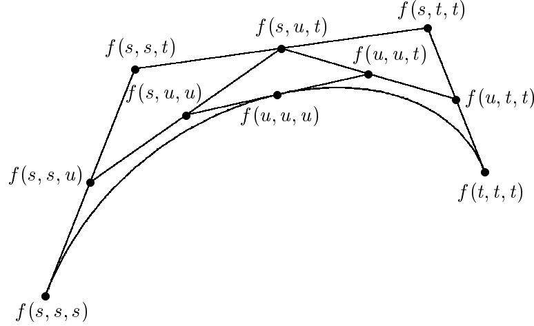
Slika 1.1: Kubična Bezier-ova krivulja: Bezier-ove točke i de Casteljau-ov algoritam
