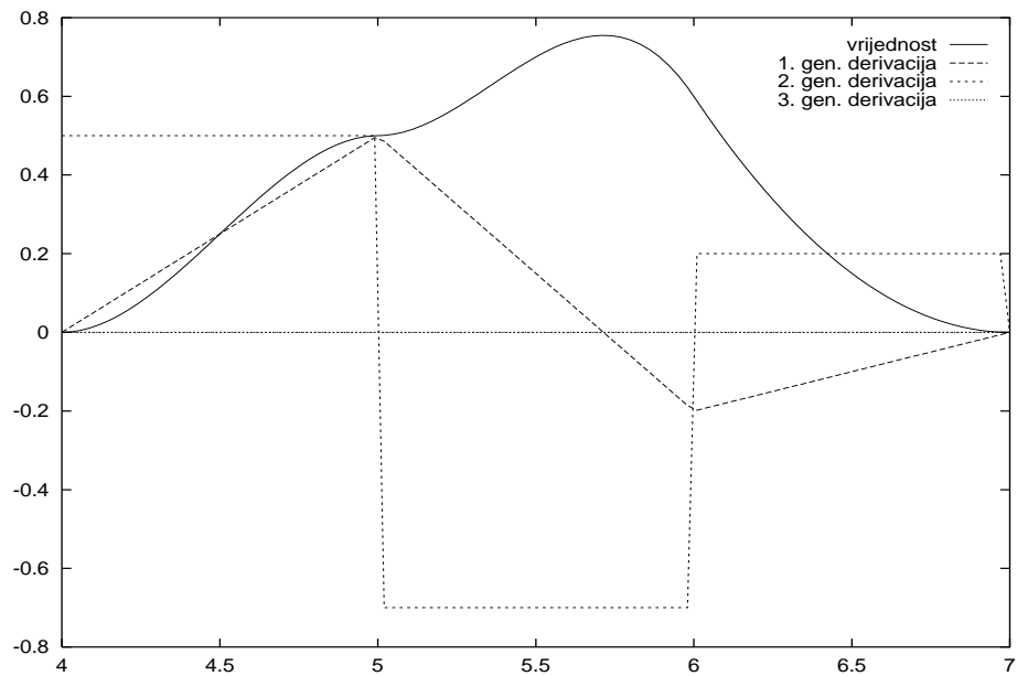
Slika 4.9: B-splajn T_4^3 i njegove obične derivacije
