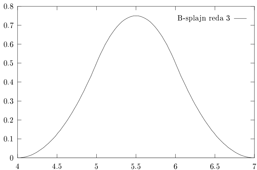
Slika 4.4: B-splajn T_4^3 za q_i = 1, i = 2, \dots, 9
