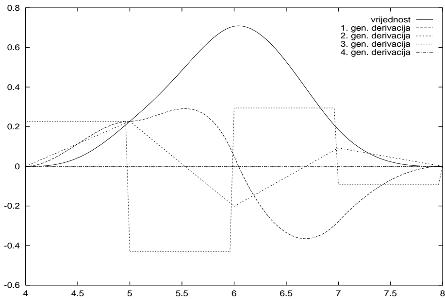
Slika 4.7: B-splajn T_4 i njegove obične derivacije
