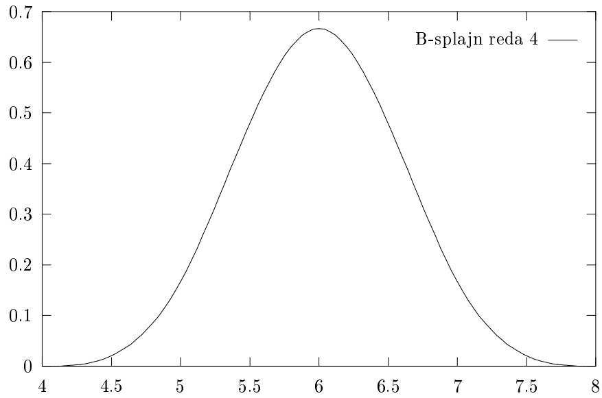
Slika 4.1: B-splajn T_4^4 za q_i = 1, i = 1, \dots, 11
