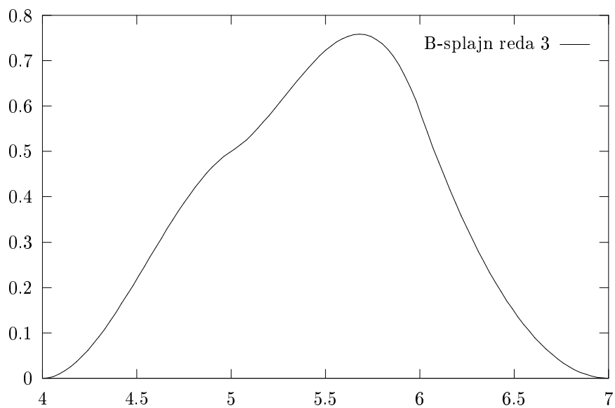
Slika 4.5: B-splajn T_4^3 za q_i = 1, i \neq 5 i q_5 = 0.1
