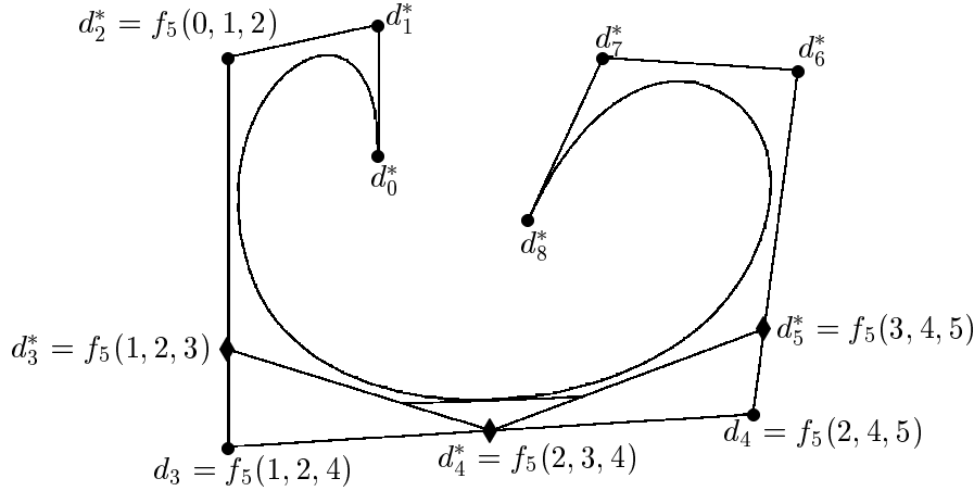
Slika 1.3: Ubacivanje novog čvora u = 3 u danu patciju T = (0, 0, 0, 0, 1, 2, 4, 5, 6, 6, 6, 6) za kubičnu B-splajn krivulju
