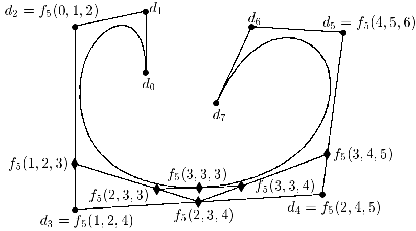
Slika 1.2: deBoor-ov algoritam za računanje vrijednosti kubične splajn krivulje nad T = (0, 0, 0, 0, 1, 2, 4, 5, 6, 6, 6, 6) u točki u = 3
