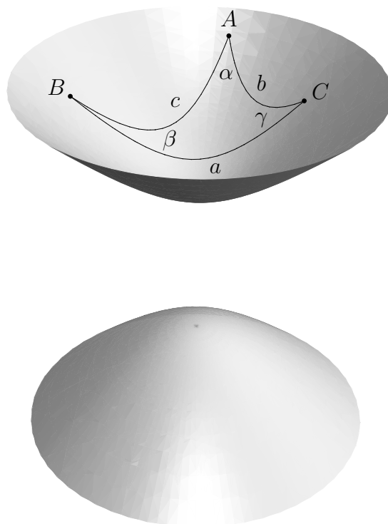
SLIKA 2. Hiperbolički trokut.
