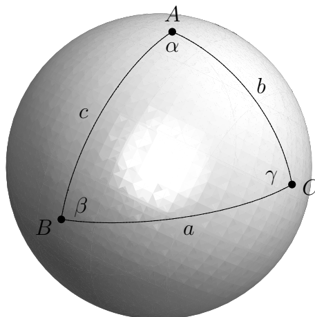
SLIKA 1. Sferni trokut.
