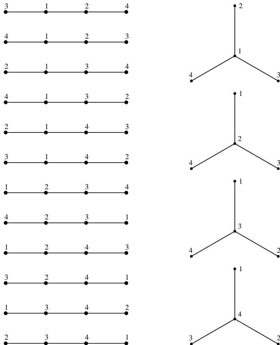
Slika 3.10: Stabla s n = 4 vrhova.
