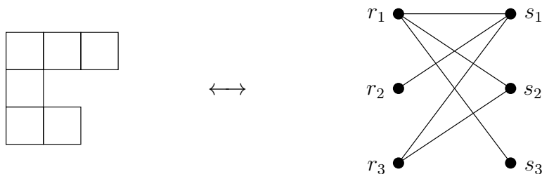
Slika 5.6: Ploča P sa slike 5.1 i odgovarajući bipartitan graf G .
