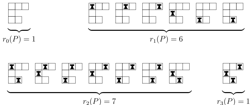
Slika 5.2: Rasporedi nenapadajućih topova na ploči P .
