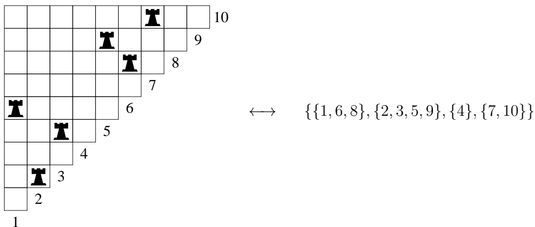
Slika 3.9: Topovska bijekcija za teorem 3.16.
