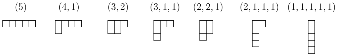
Slika 3.3: Ferrersovi dijagrami particija broja 5.
