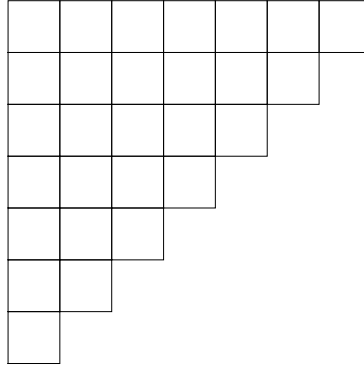
Slika 3.7: Ploča \Delta_8 .
