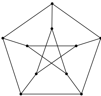
Slika 1.4: Petersenov graf.
