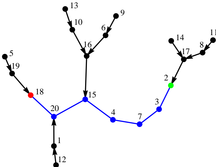
Slika 3.11: Primjer kralježnjaka s n = 20 vrhova.
