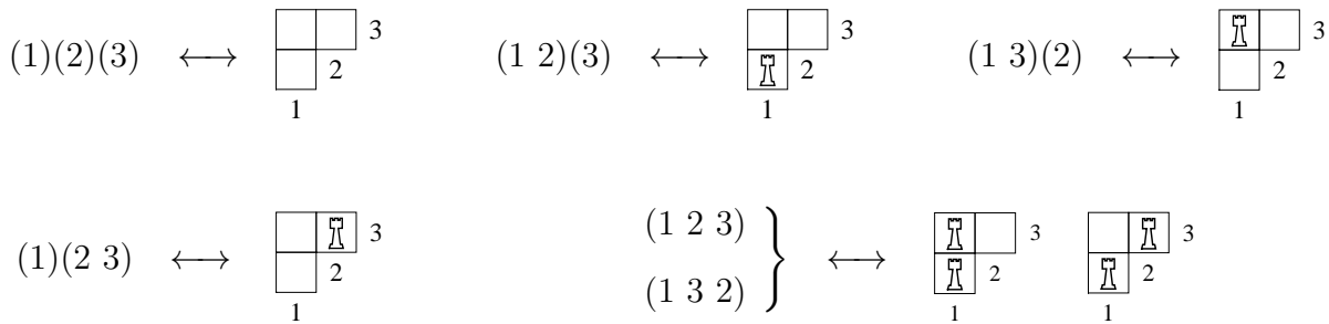
Slika 4.2: Sloperovska bijekcija za n = 3 .
